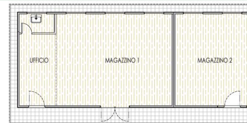
NUOVO MAGAZZINO - PIANTA
